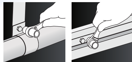
ディープボックスタイプ
