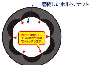
機能特徴図
