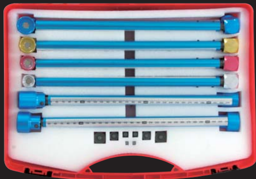
サービスホールゲージ用 アタッチメント 6・10・15・20mm
